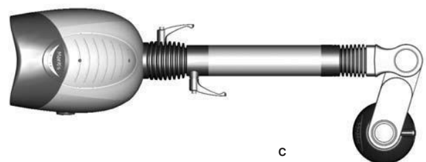
Verlengde arm met extra verlangstuk weggedraaid: Bereik C = 639.0mm
