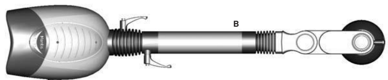
Verlengde arm met extra tussenstuk bereik B = 847.5mm
